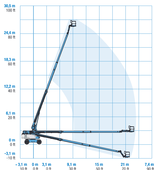
ARBEITSDIAGRAMM S™-85
