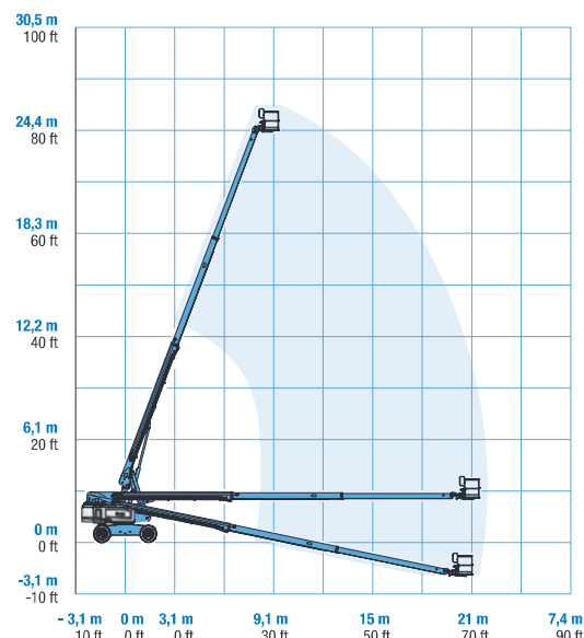
ARBEITSDIAGRAMM S™-85
